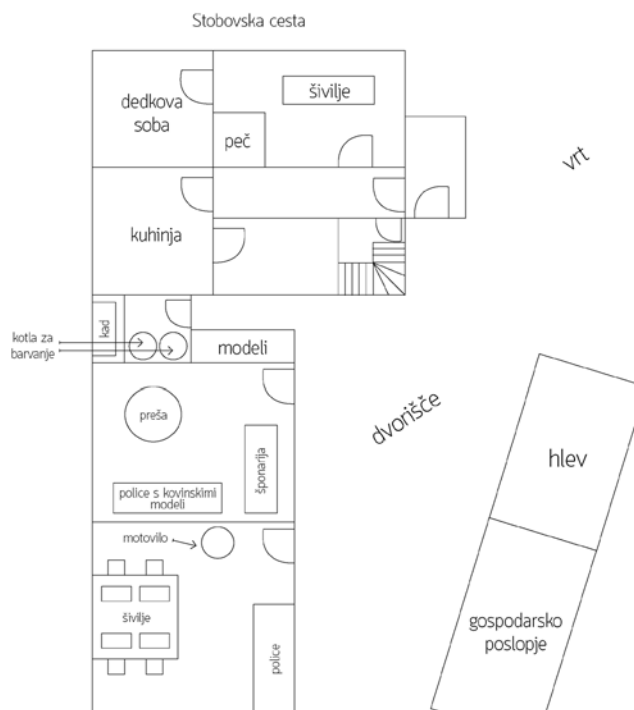
Skica 1: Razporeditev opreme v Koširjevih delavnicah (risali: T. Jeras in A. Sokler).
